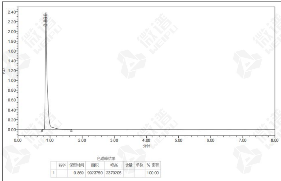
图 1 样品经稀释 HPLC 测试结果
